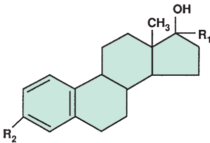
Estradiol
