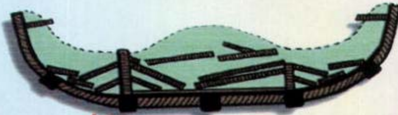
رسم تفصيلي لهيكل السفينة من الداخل
